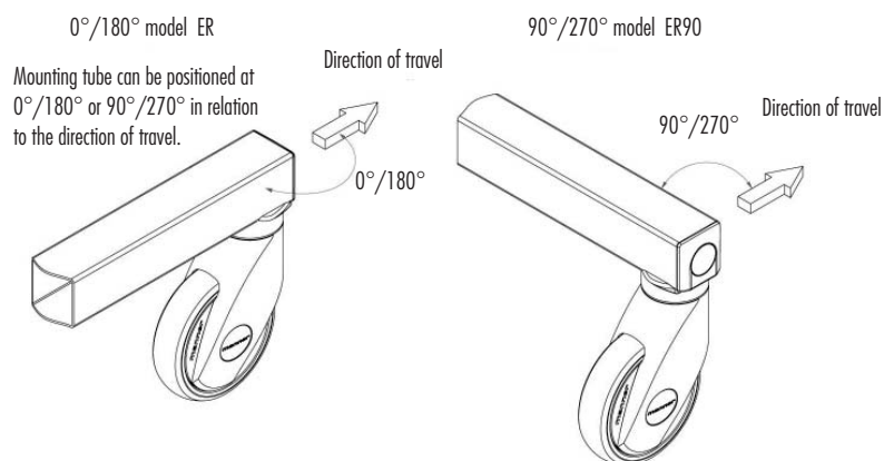
Monteringsmuligheder for e-SMART hjul med retningsspærrer.
