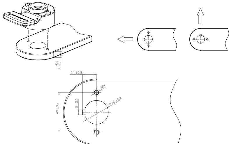
SMART-hjul monteringsmål.
